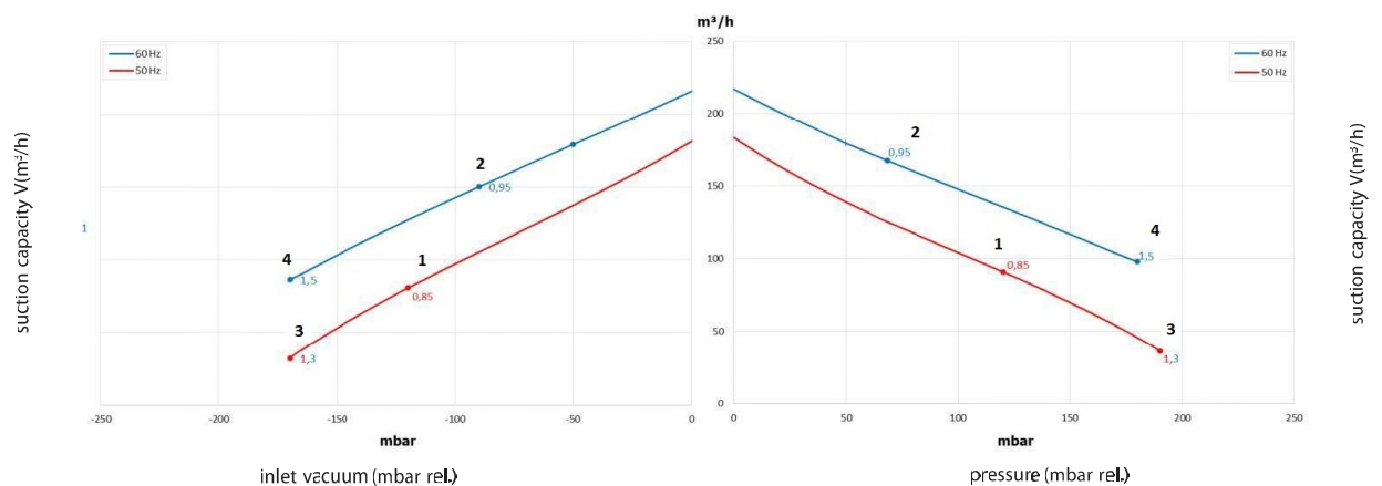
Zuigzijde / EXHAUST
