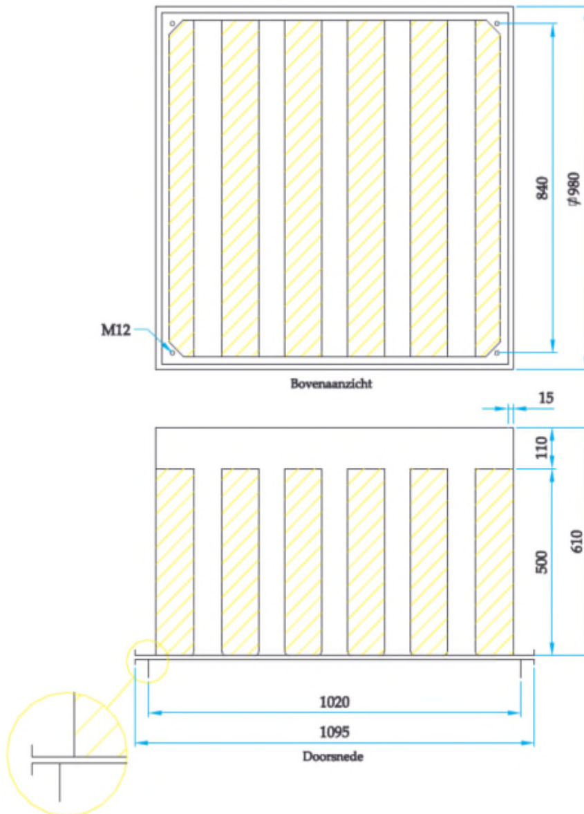
Bovendakse geluiddemper Verzinkt plaatstaal
